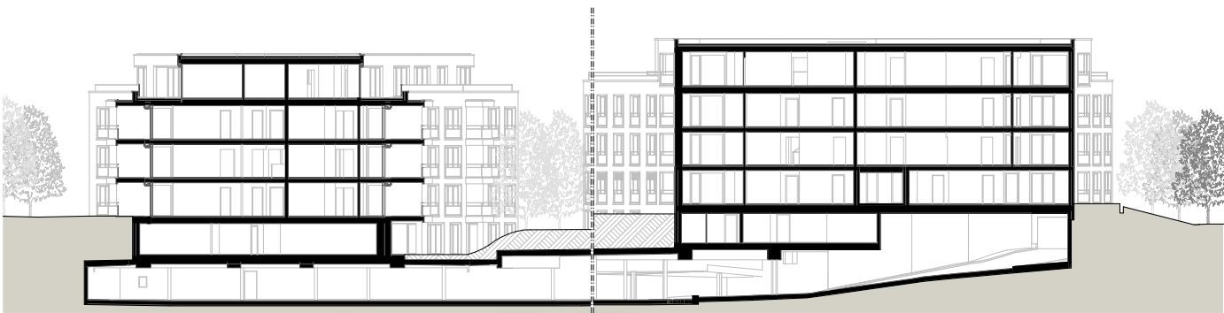
Schnitt A 1:500
