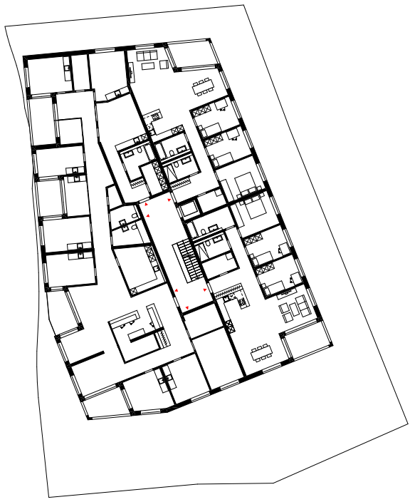
⌚ Grundriss 1. – 3. OG 1:500
