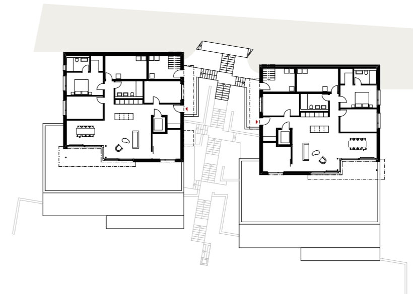
Ebene 3 1:500
