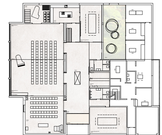
Grundriss Erdgeschoss 1:500
