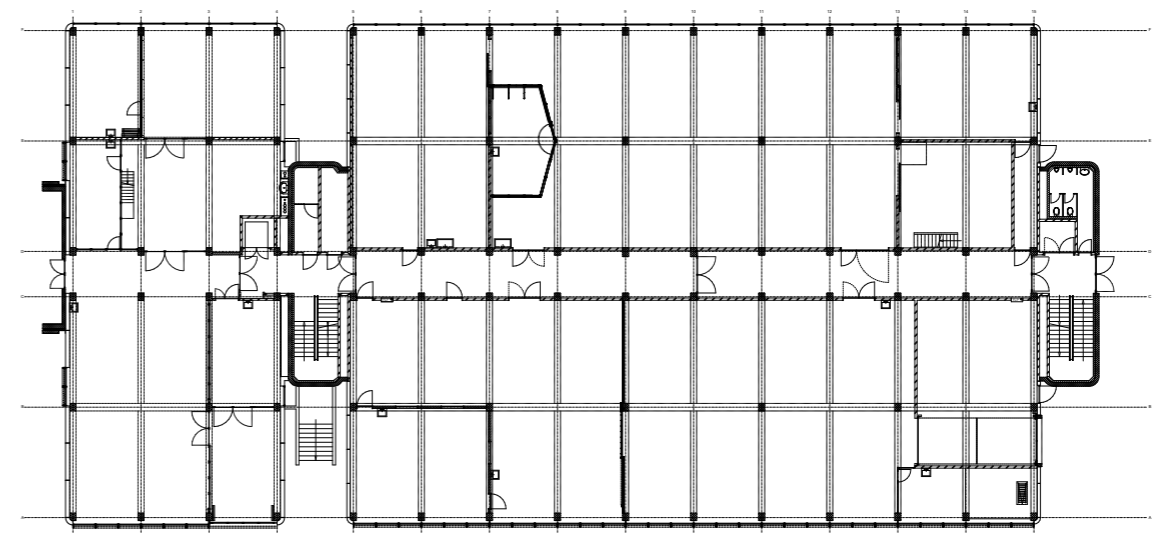
Grundriss Erdgeschoss 1:500
